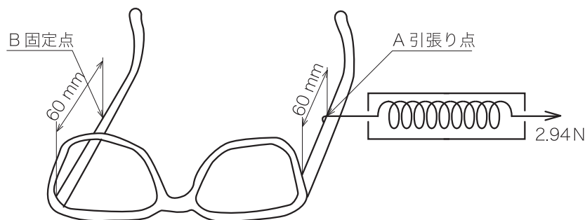
図 10－把持性試験（第 1 試験）（図は一例を示す。）
