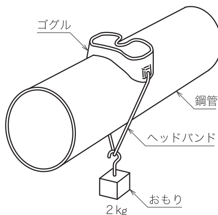
図 12—ヘッドバンド取付部の強度試験 (図は一例を示す。)
