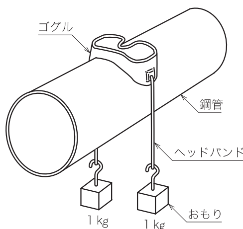
図 13—安全帽取付形用ヘッドバンド取付部の強度試験 (図は一例を示す。)
