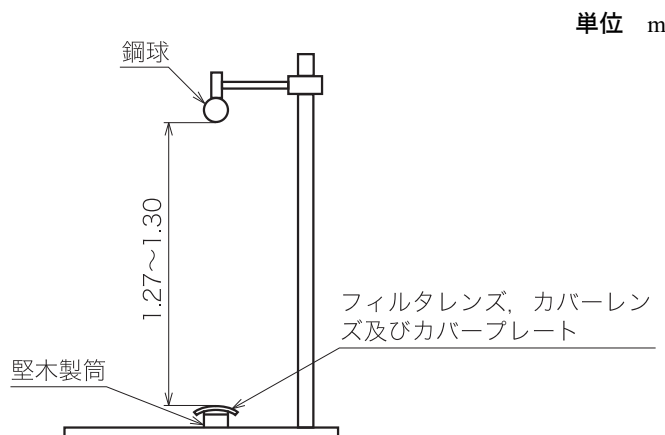
図 2—耐衝撃性試験装置 (図は一例を示す。)
